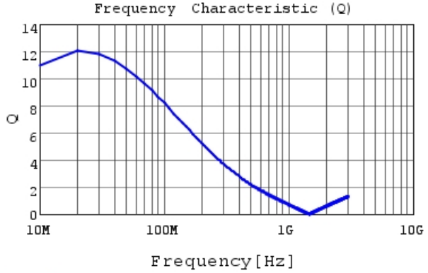
LQW15CNR22K1Z Q
