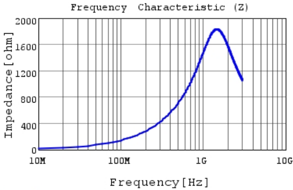
LQW15CNR22K1Z |Z|
