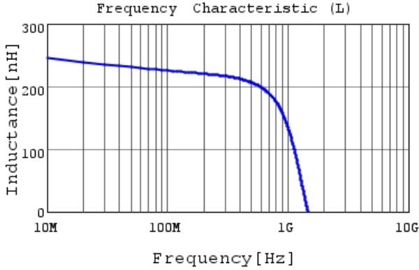
LQW15CNR22K1Z L
