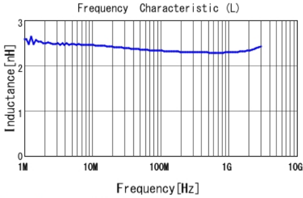
LQW15AN2N3C8Z L
