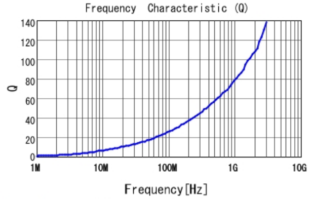
LQW15AN2N3C8Z Q
