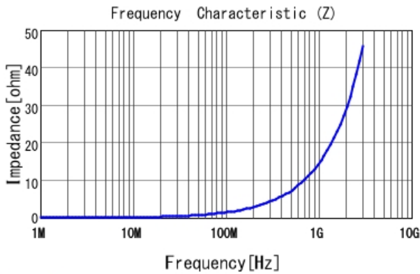
LQW15AN2N3C8Z |Z|
