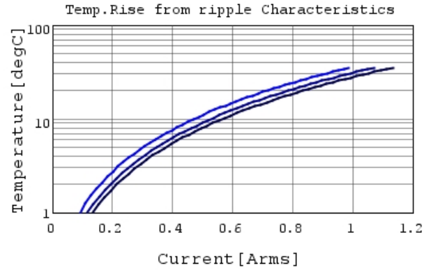
GRT033C81E104KE01 Temp.rise — 400kHz —
