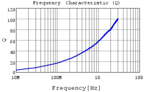
LQW15AN5N8C00 Q
