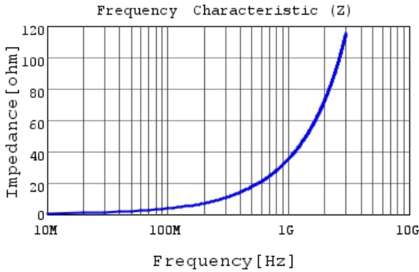
LQW15AN5N8C00 |Z|
