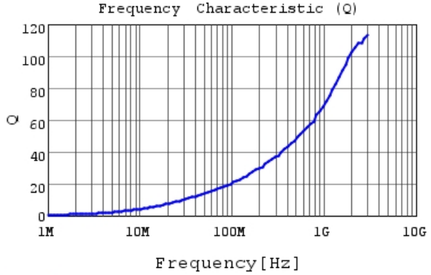
LQW15AN2N9B80 Q
