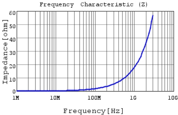
LQW15AN2N9B80 |Z|
