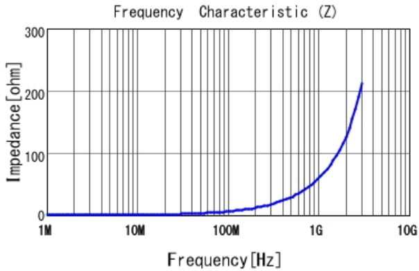
LQW15AN9N5J80 |Z|
