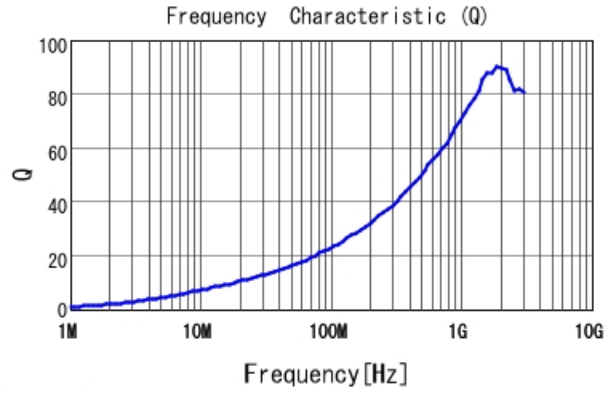
LQW15AN9N5J80 Q
