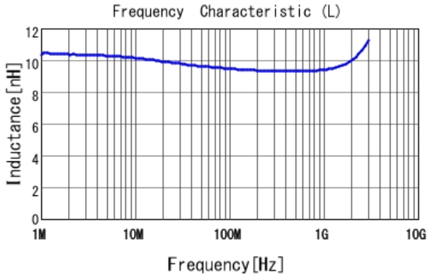
LQW15AN9N5J80 L
