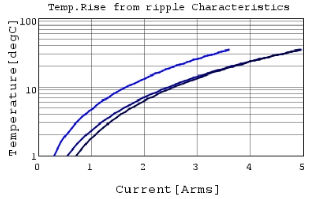
GRM188C81C106MA73 Temp.rise — 80kHz
