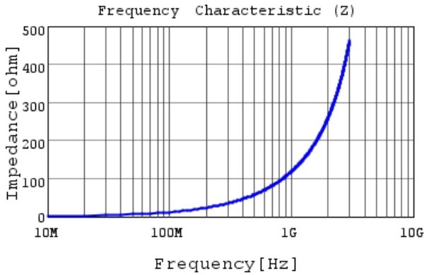
LQW15AN19NJ0Z |Z|
