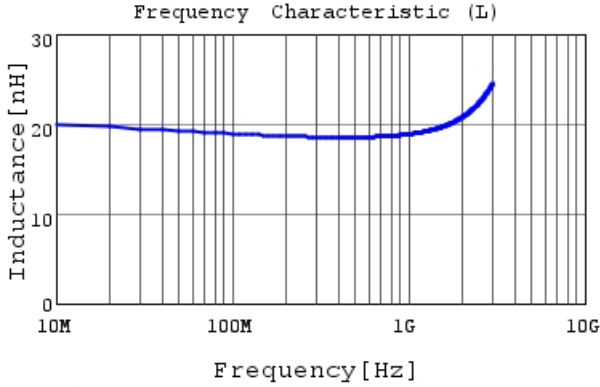
LQW15AN19NJ0Z L
