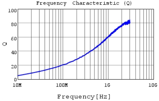
LQW15AN19NJ0Z Q
