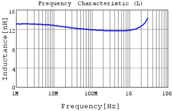
LQW15AN12NG80 L
