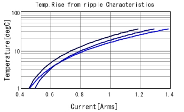
GJM1555C1H200JB01 Temp. rise — 500MHz — 700I
