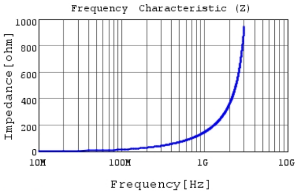
LQP02HQ22NH02 |Z|
