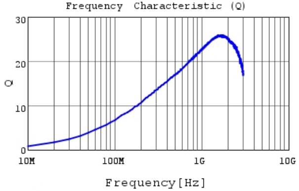
LQP02HQ22NH02 Q
