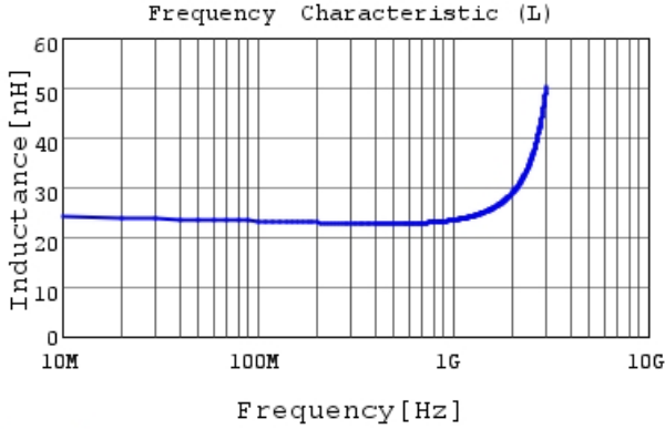
LQP02HQ22NH02 L
