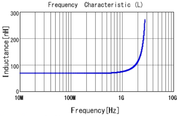
LQW15AN68NG00 L
