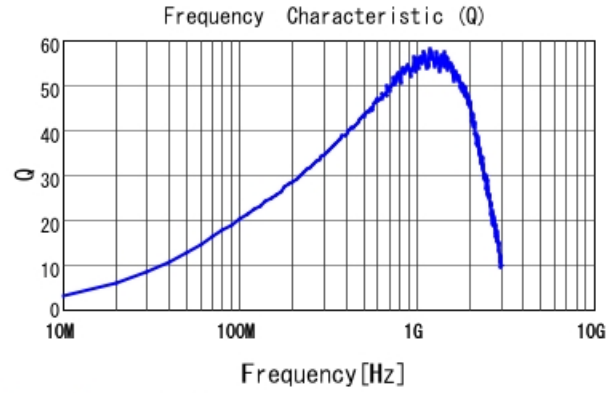
LQW15AN68NG00 Q
