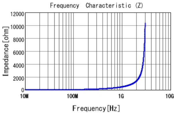
LQW15AN68NG00 |Z|
