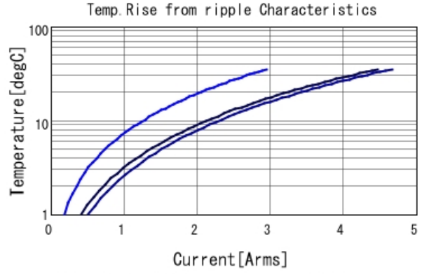
GRM219R61H225KE15 Temp. rise — 100kHz — 500
