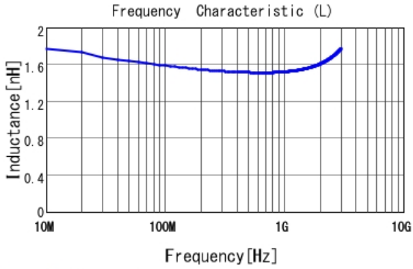
LQG15HH1N6C02 L
