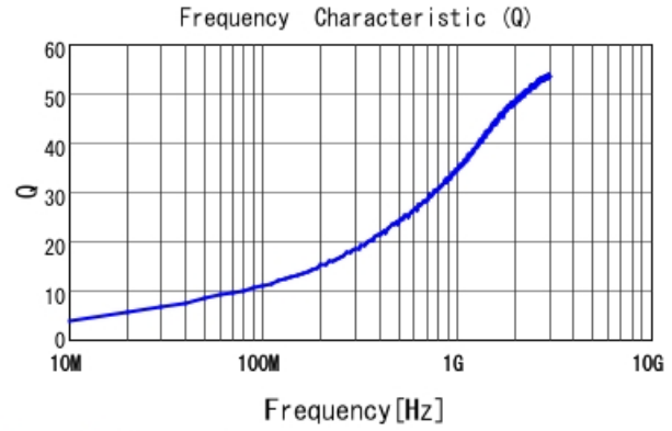
LQG15HH1N6C02 Q
