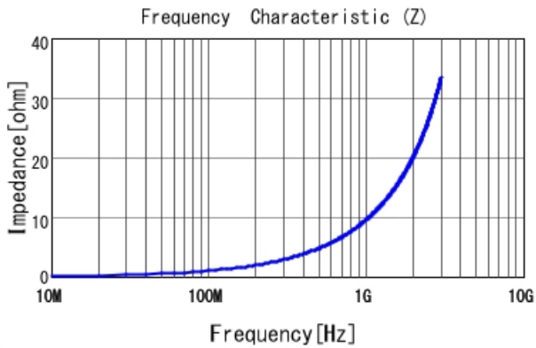
LQG15HH1N6C02 |Z|
