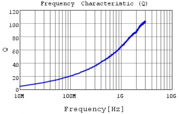
LQW15AN7N3J00 Q
