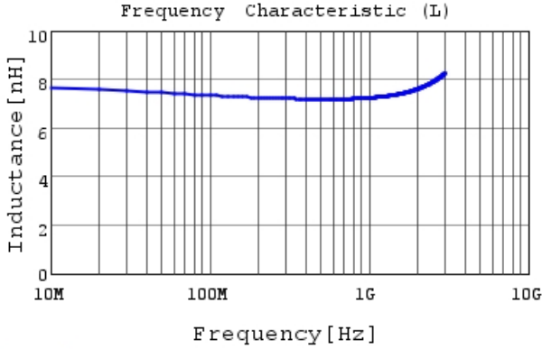
LQW15AN7N3J00 L
