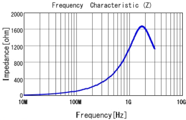
LQW15CAR18J00 |Z|
