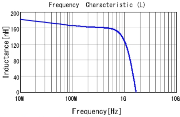
LQW15CAR18J00 L
