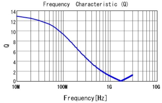
LQW15CAR18J00 Q
