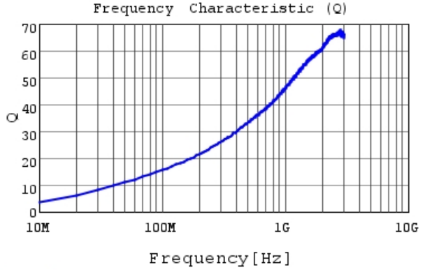
LQW04AN10NJ00 Q
