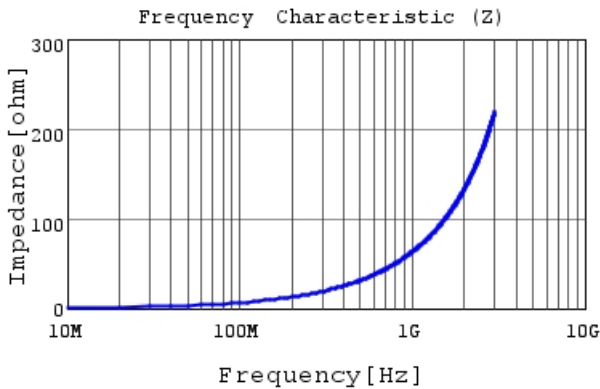
LQW04AN10NJ00 |Z|
