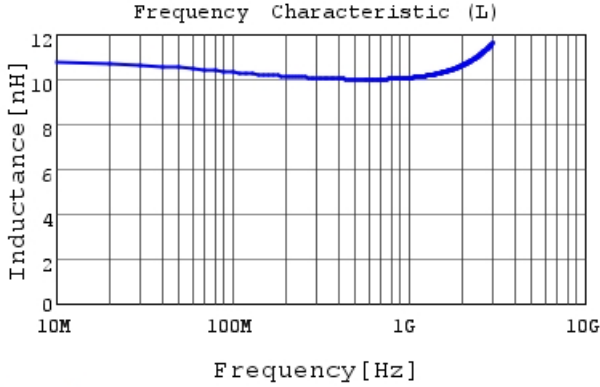
LQW04AN10NJ00 L
