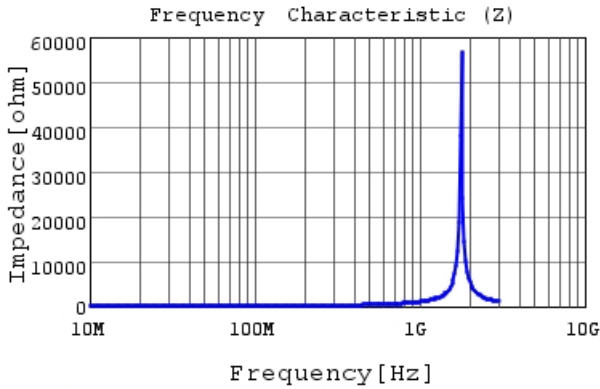
LQW18ANR12J8Z |Z|
