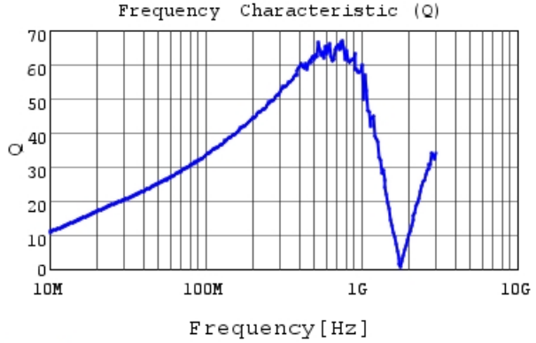
LQW18ANR12J8Z Q
