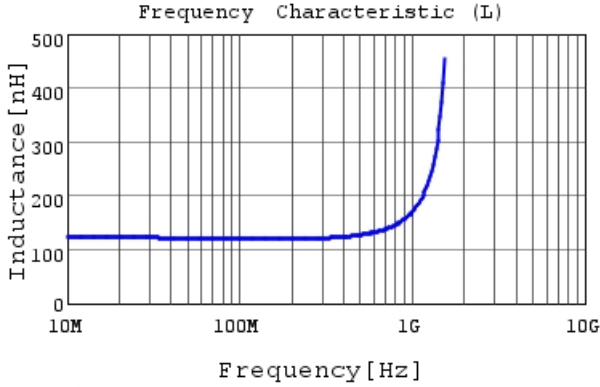
LQW18ANR12J8Z L
