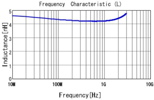
LQP03HQ4N2B02 L
