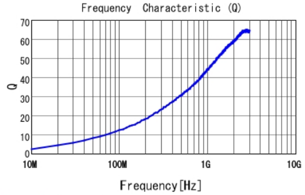
LQP03HQ4N2B02 Q
