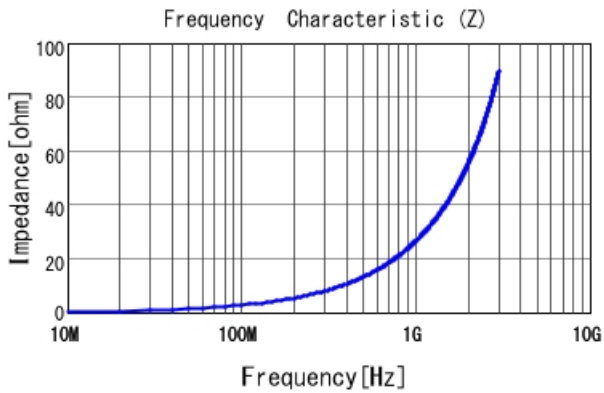
LQP03HQ4N2B02 |Z|
