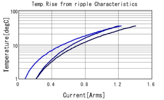
GRM155R61E104KA87 Temp. rise — 400kHz — 800kHz
