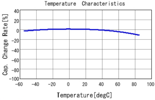
GRM155R61A474ME15 C-Temp. capchange, DCO. 0V, ACO. 5
