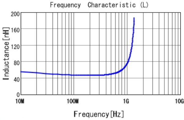
LQG15HN47NH02 L
