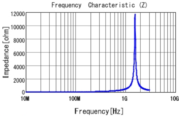
LQG15HN47NH02 |Z|
