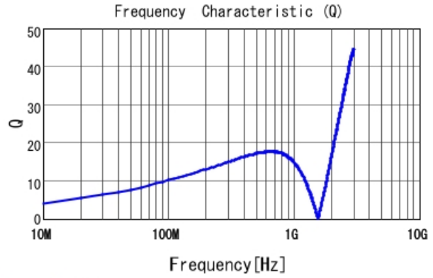
LQG15HN47NH02 Q
