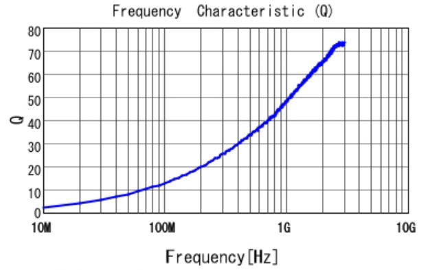
LQP03HQ3N2B02 Q
