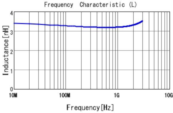
LQP03HQ3N2B02 L
