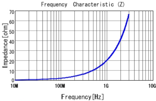
LQP03HQ3N2B02 |Z|
