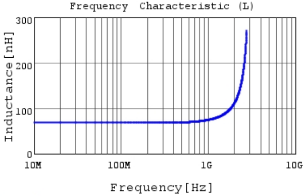
LQW15AN68NJ00 L
