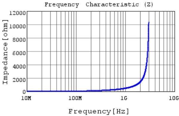
LQW15AN68NJ00 |Z|
