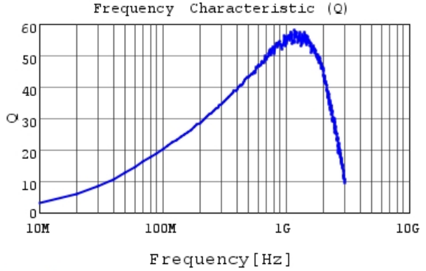
LQW15AN68NJ00 Q
