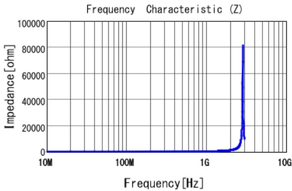
LQW15AW53NG80 |Z|
