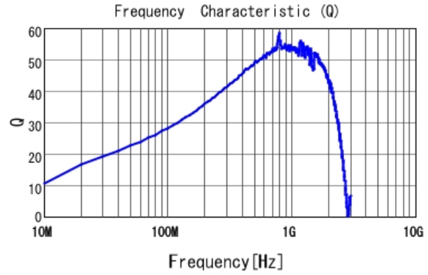
LQW15AW53NG80 Q
