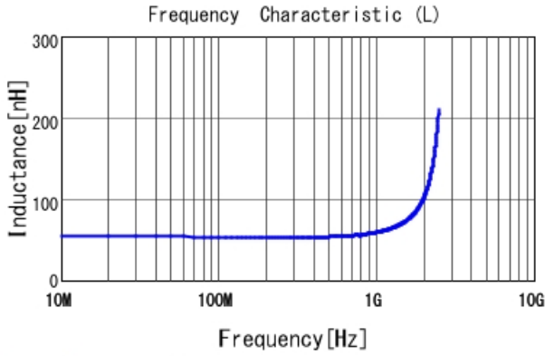
LQW15AW53NG80 L
