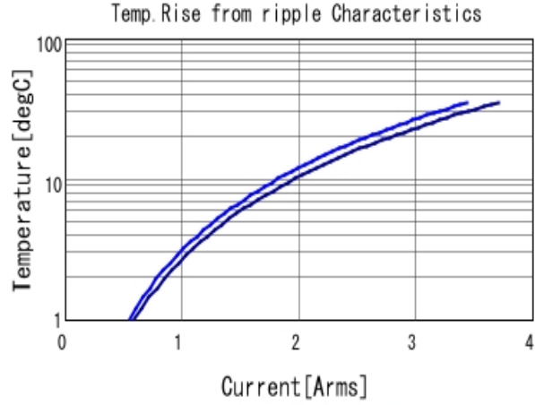
GRM219R7YA105MA12 Temp. rise ■ 500kHz ■ 1MHz
