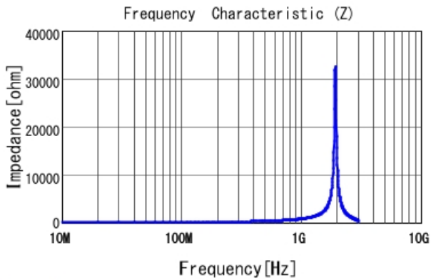
LQW15ANR10J00 |Z|
