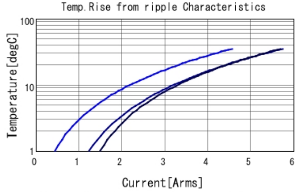
GRM21BC80J226ME51 Temp. rise — 80kHz — 400kHz
