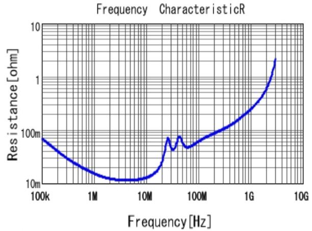
■ GRJ32DR72E224KWJ1 R DCOV, 25degC
