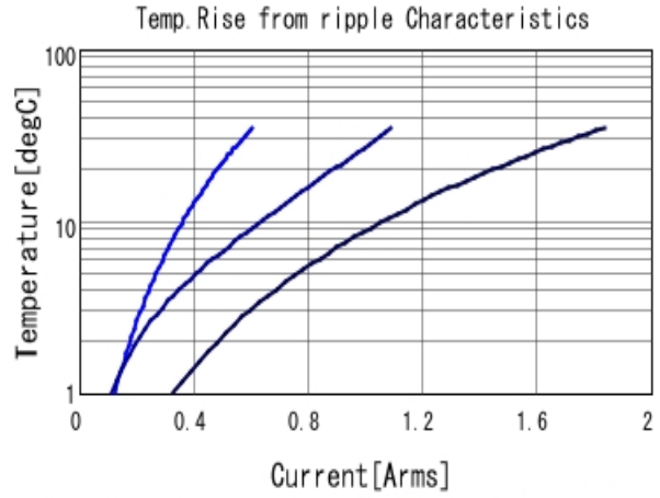
GRJ32DR72E224KWJ1 Temp. rise ■ 30kHz ■ 100kHz ■ 300kHz
