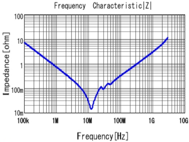
■ GRJ32DR72E224KWJ1 |Z| DCOV, 25degC
