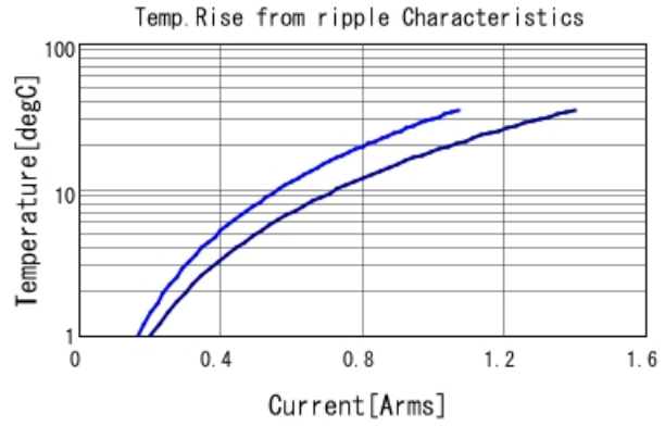
GRM155R61H104ME14 Temp. rise — 500kHz — 1MHz
