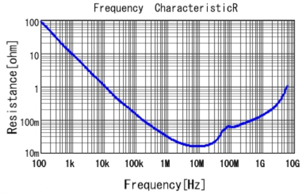
GRM155R61H104ME14 R DCOV, 25degC
