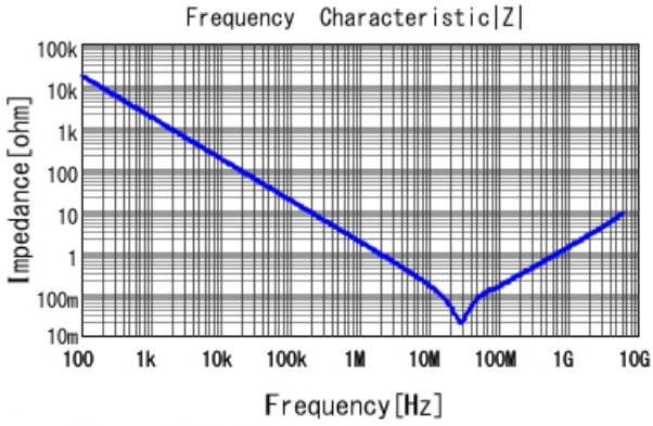
GRM155R61H104ME14 |Z| DCOV, 25degC
