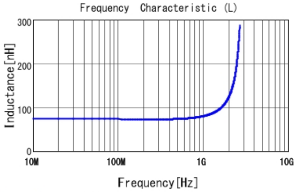
LQW15AN72NG00 L
