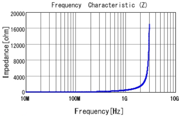
LQW15AN72NG00 |Z|
