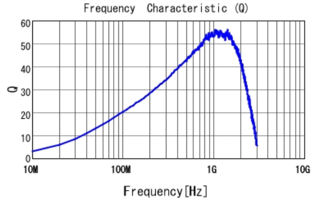
LQW15AN72NG00 Q
