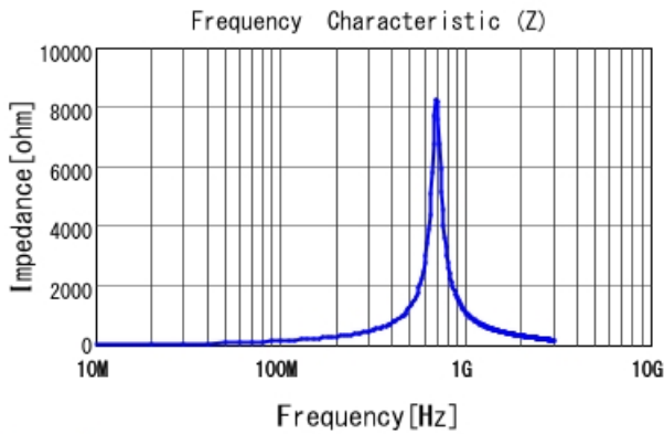
LQP03TNR22H02 |Z|
