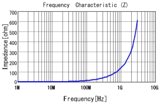
LQW15AN22NJ8Z |Z|
