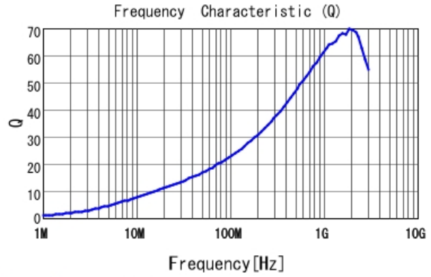
LQW15AN22NJ8Z Q
