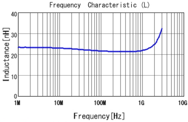
LQW15AN22NJ8Z L
