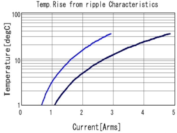
GRM21BB10J225KA01 Temp. rise ■ 100kHz ■ 500kHz ■ 1MHz
