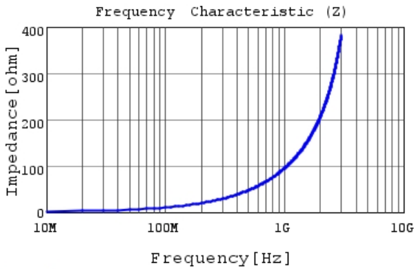
LQP02TQ15NH02 |Z|
