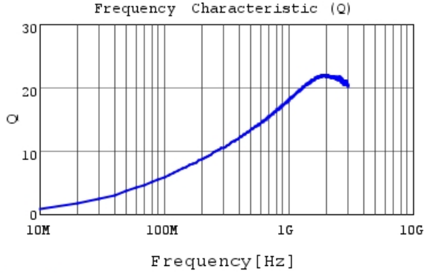
LQP02TQ15NH02 Q
