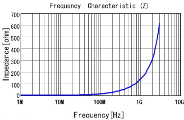
LQW15AN22NJ80 |Z|
