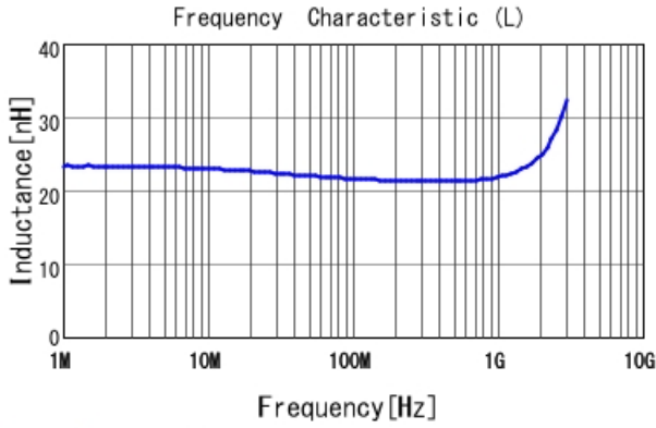
LQW15AN22NJ80 L
