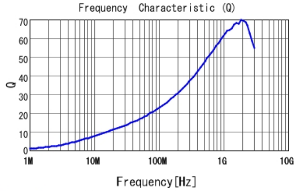
LQW15AN22NJ80 Q
