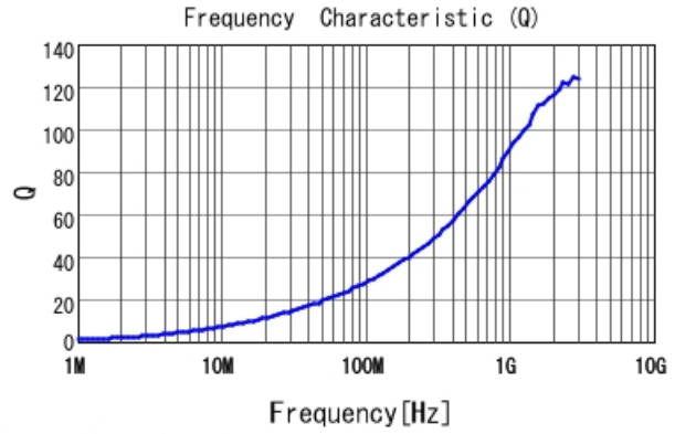
LQW18AN9N5C80 Q
