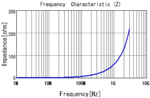
LQW18AN9N5C80 |Z|
