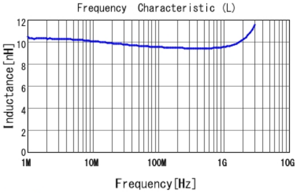
LQW18AN9N5C80 L
