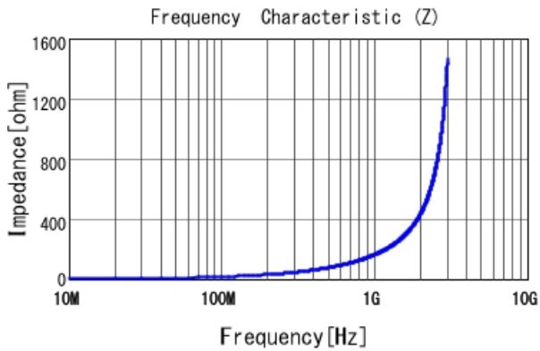
LQW18AS24NG0Z |Z|
