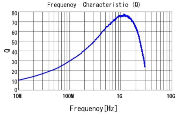
LQW18AS24NG0Z Q
