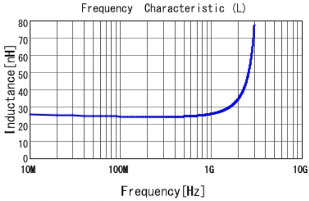
LQW18AS24NG0Z L
