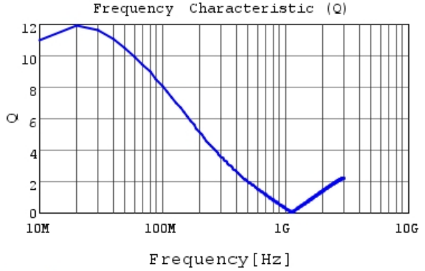
LQW15CNR27J1Z Q
