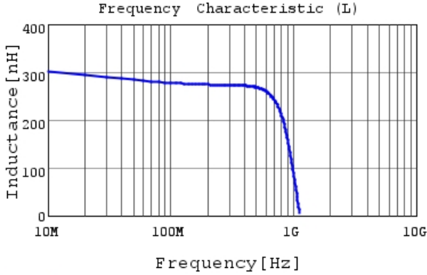
LQW15CNR27J1Z L
