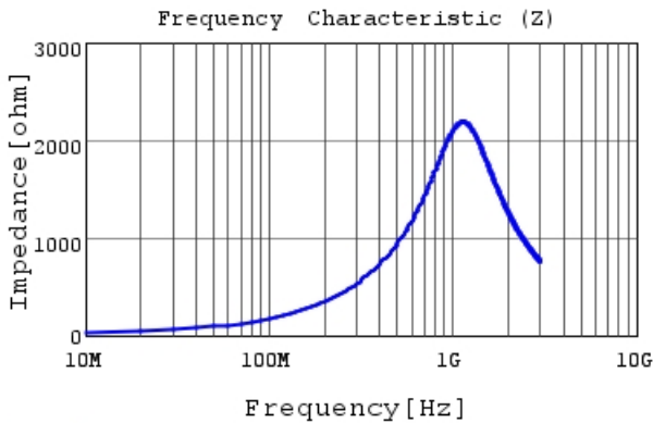
LQW15CNR27J1Z |Z|
