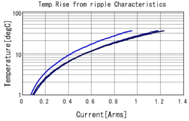
GCM155R71C154KE02 Temp. rise — 400kHz — 800
