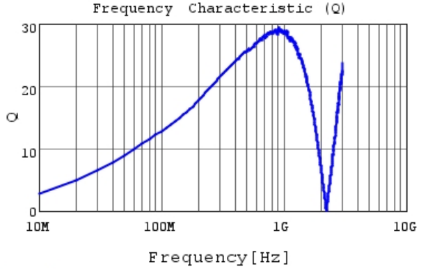
LQP03HQ47NH02 Q
