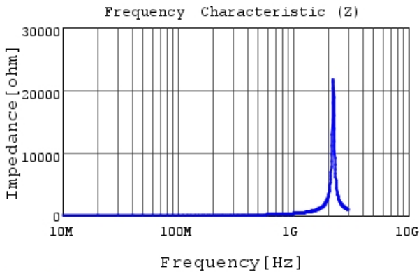
LQP03HQ47NH02 |Z|
