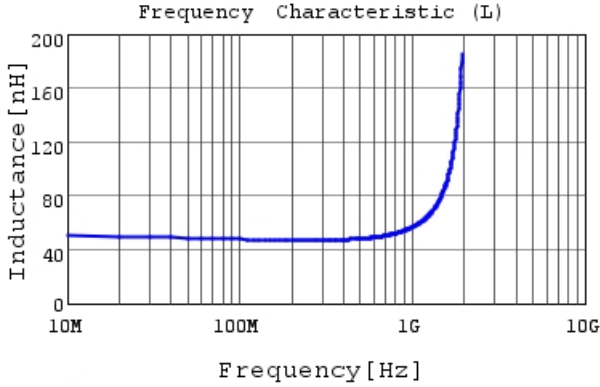
LQP03HQ47NH02 L
