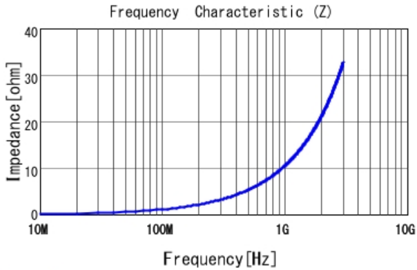
LQW15AN1N8C0Z |Z|
