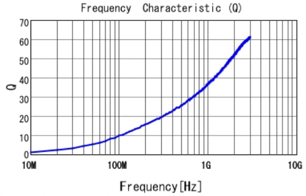
LQW15AN1N8C0Z Q
