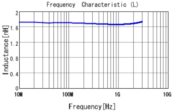
LQW15AN1N8C0Z L
