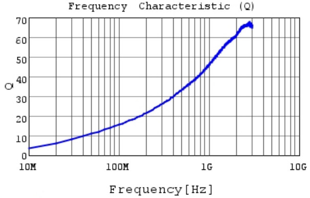
LQW04AN10NH00 Q
