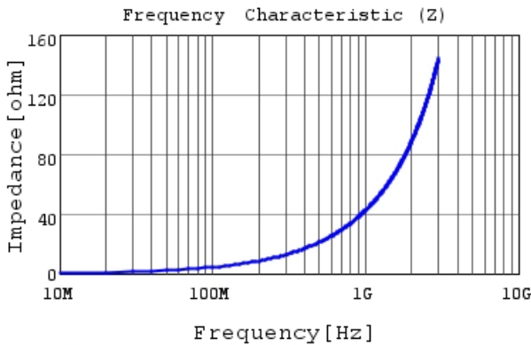
LQW15AN6N8J00 |Z|
