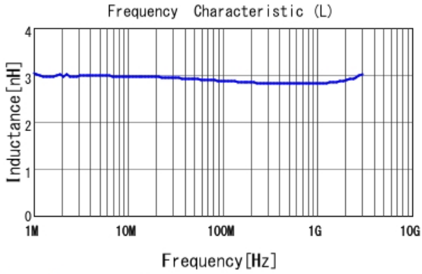
LQW15AN2N9B8Z L
