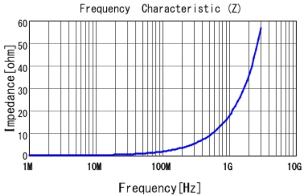
LQW15AN2N9B8Z |Z|
