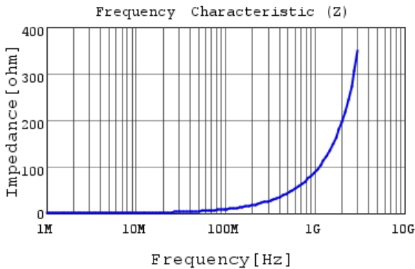
LQW15AN14NJ80 |Z|
