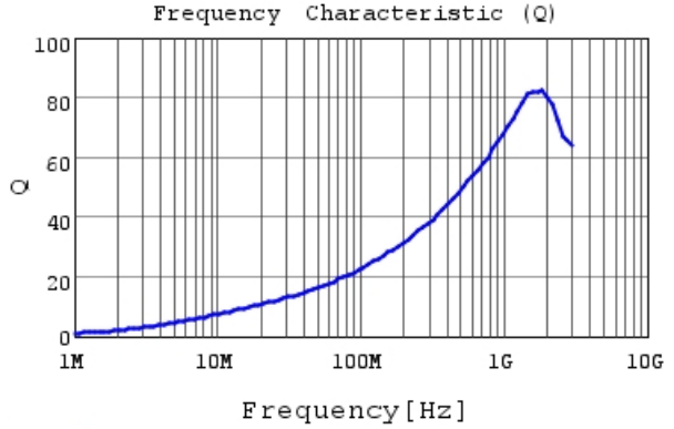
LQW15AN14NJ80 Q
