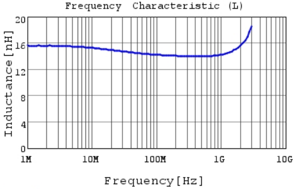
LQW15AN14NJ80 L
