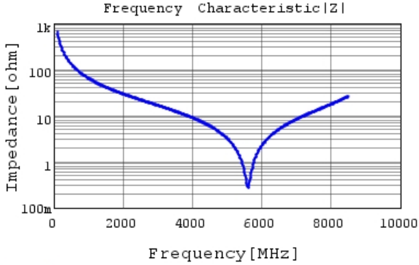
GCQ1555C1H2R4WB01 |Z| DC0V, 25degC
