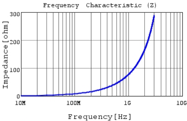
LQW15AN12NH0Z |Z|
