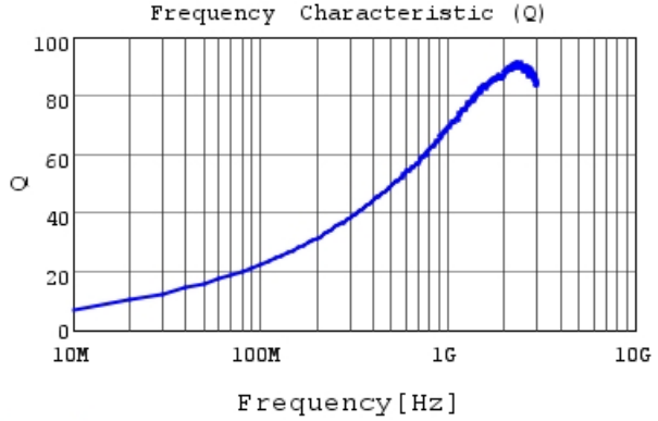
LQW15AN12NH0Z Q
