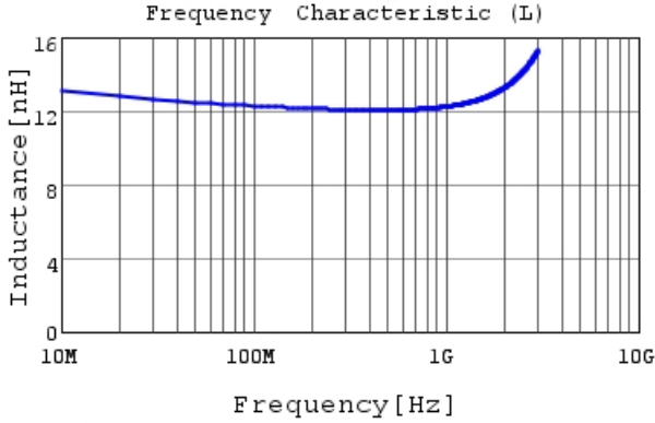
LQW15AN12NH0Z L
