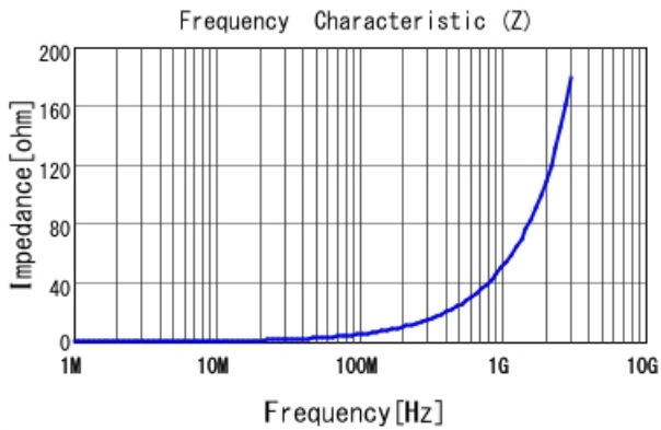
LQW18AN8N2C80 |Z|
