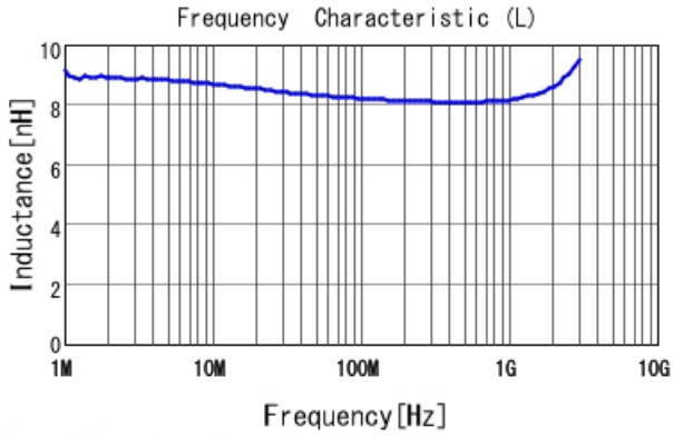
LQW18AN8N2C80 L
