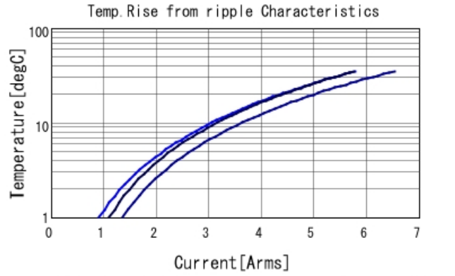
GRM32ER61C476ME15 Temp. rise — 60kHz — 300kHz
