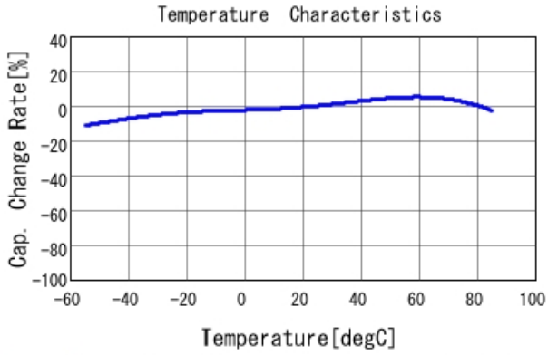
GRM32ER61C476ME15 C-Temp. capchange, DCO. 0V, ACO. 5
